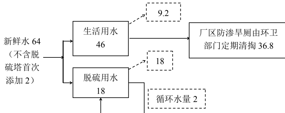
图 2-2 项目排水水平衡图 (单位 \text{m}^3/\text{a} )
