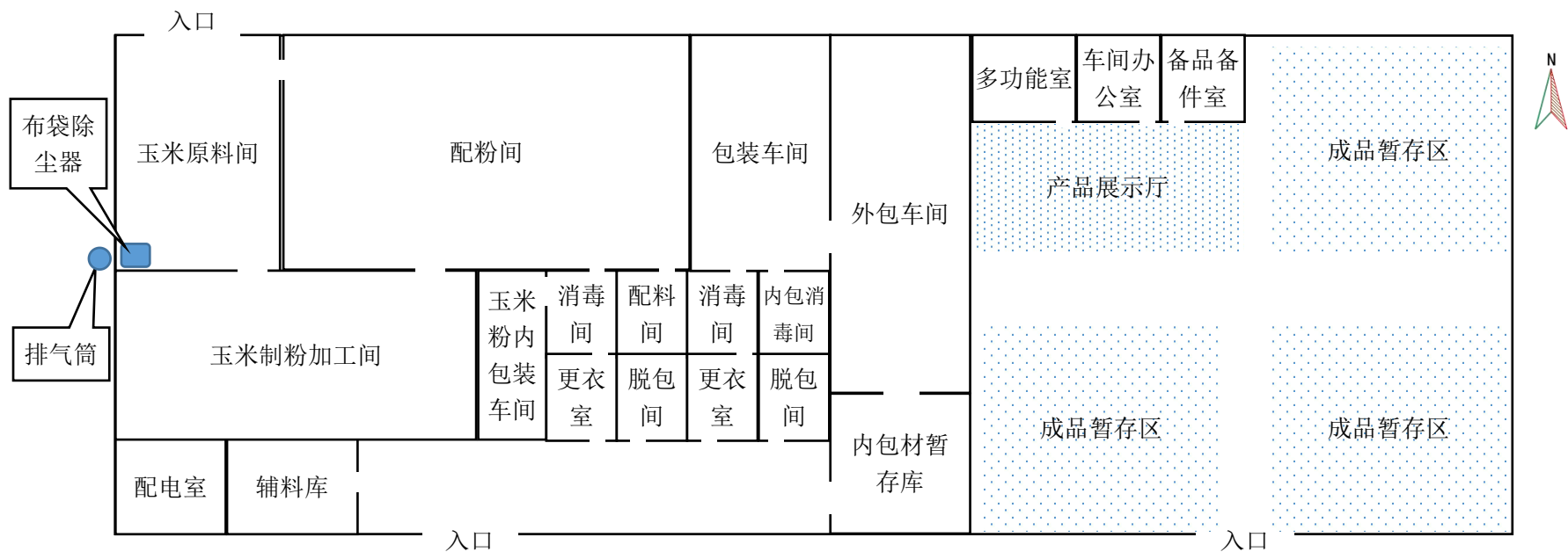
附图 4 平面布置图 1: 300
