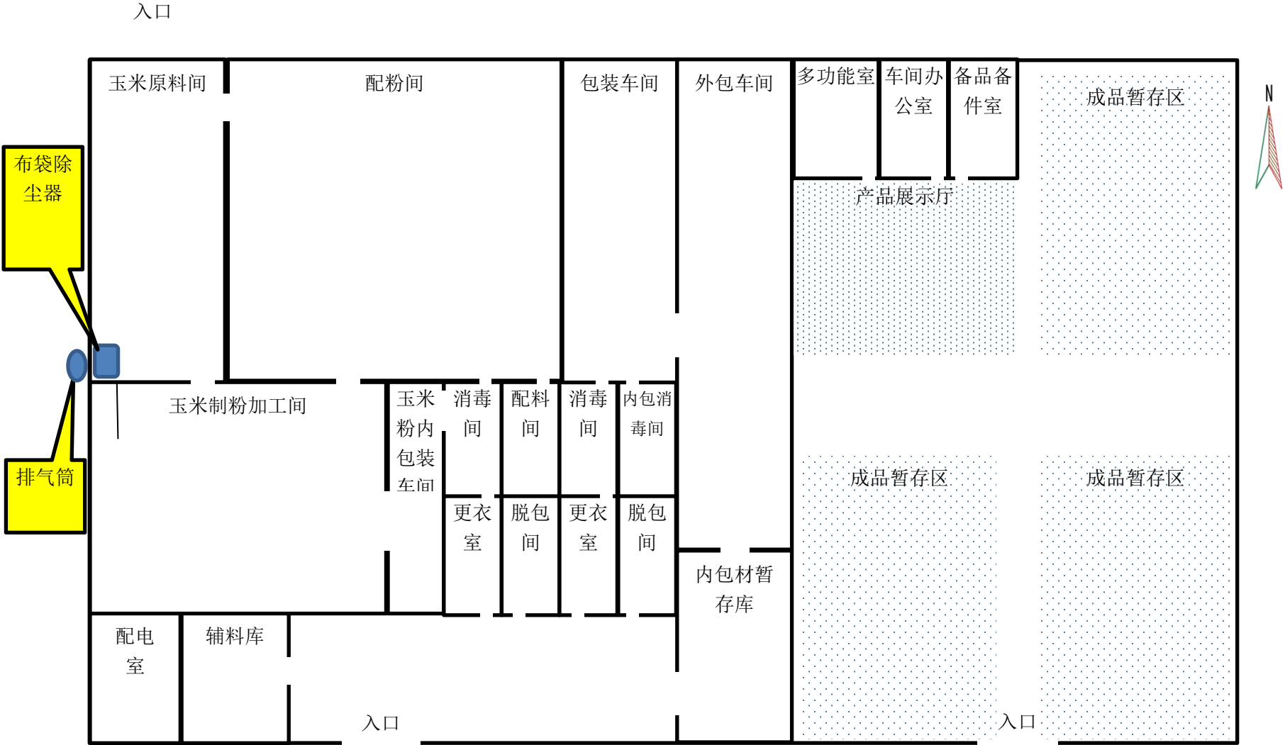
张家口图隆元食品有限公司玉米深加工项目污染治理图
