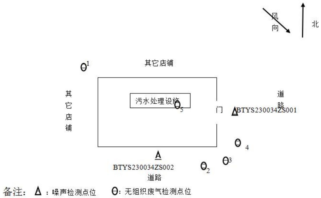
图 6-1 检测点位图
