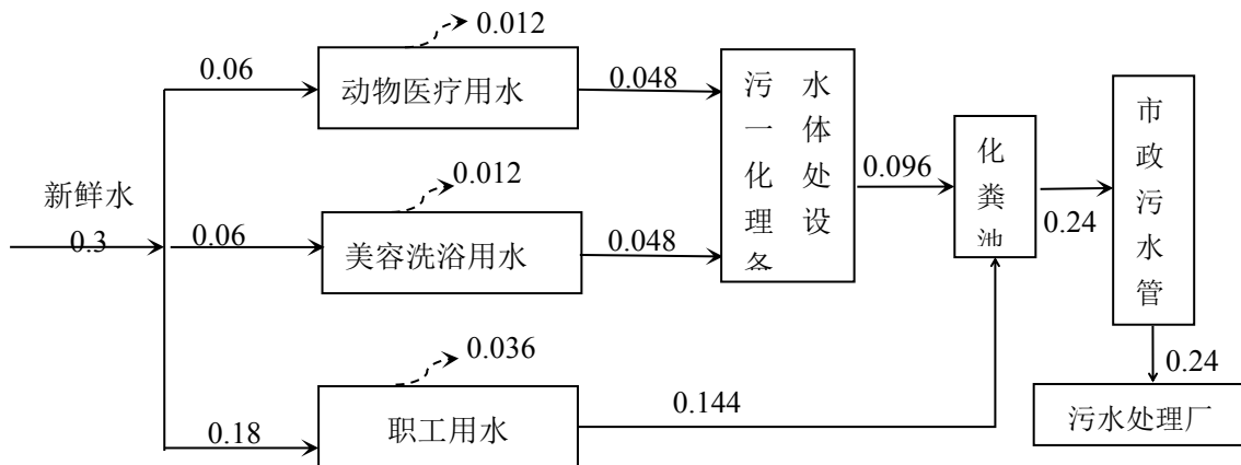
图 2-2 水平衡图 (m 3 /d)
